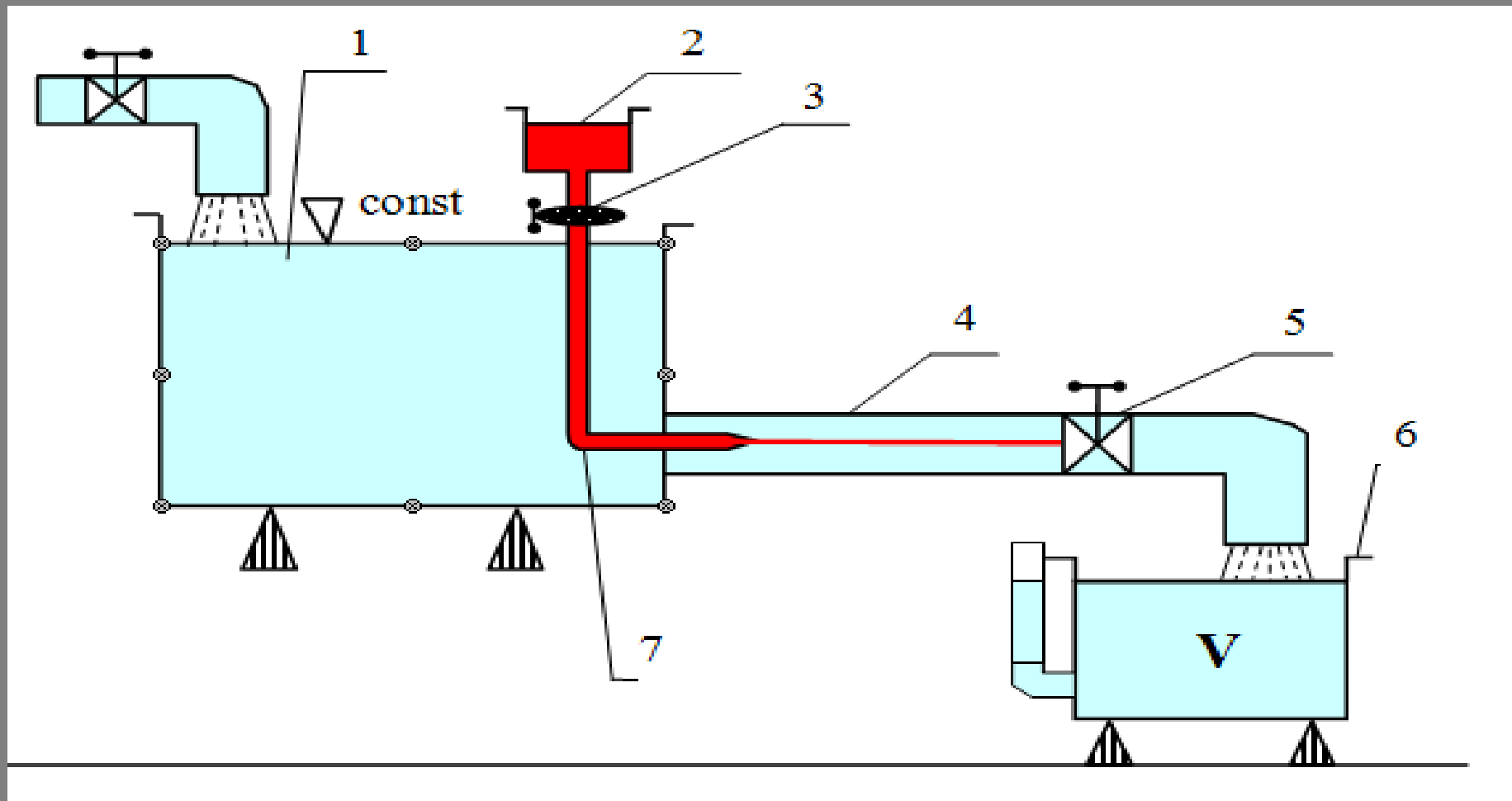
6.2 – rasm. Reynolds tajribasi.
